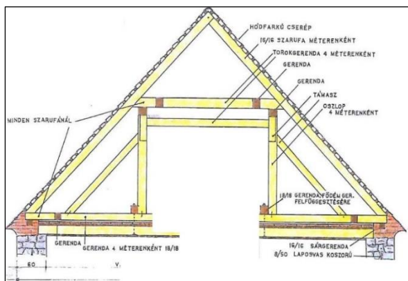
Cselédlakások tetőszerkezete. (szerkesztette, rajzolta: Heffler László)
