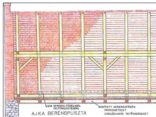
Cselédlakások tetőszerkezete. (szerkesztette, rajzolta: Heffler László)
